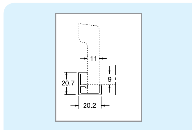
ECET Edge Trim Profile
