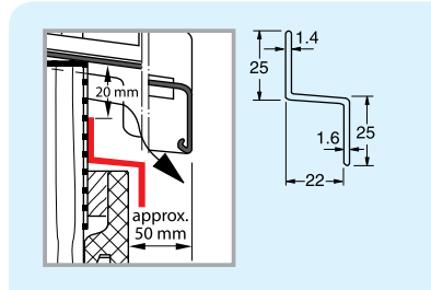
ECZP Z Profile
